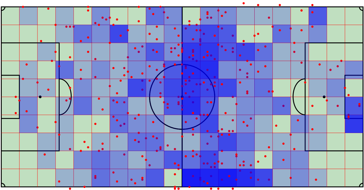
Рис.2 Пример тепловой карты выполнения ТТД PASS командой гостей
